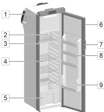
Afb. 147: 12 V compressor-koelkast
