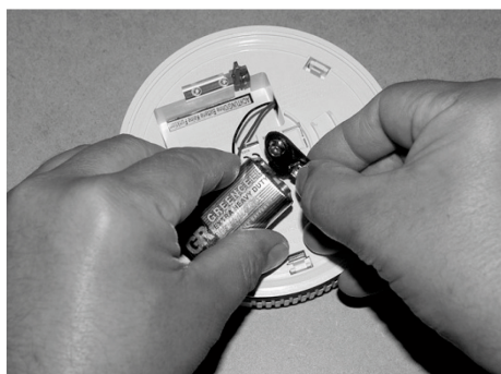
Afb. 162: Blokbatteij vervangen
