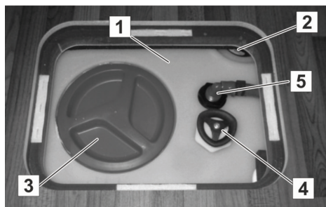
Afb. 81: Plaatsing onder de vloer
