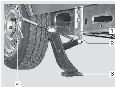
Afb. 199: Wagenkrik, AL-KO
