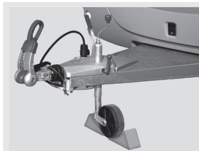
Afb. 196: Steunwiel borgen
