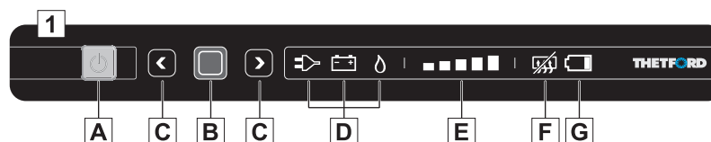
Afb. 190: LED-bedieningspaneel
