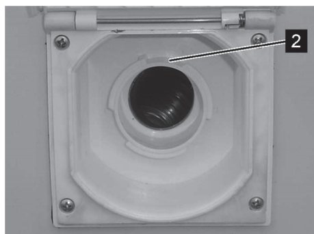
Afb. 103: Vultuit voor vers water, open
