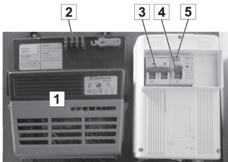
Afb. 60: Omvormer (netvoeding) (1) en zekeringautomaten
