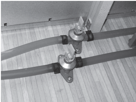
Afb. 99: Aftapkranen open
