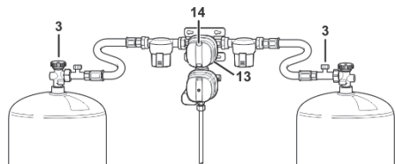
Afb. 112: Gasdrukregelset
