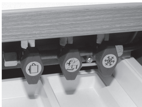
Afb. 78: Snelsluitkranen
