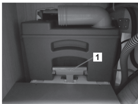
Afb. 175: Fecaliëntank in het afvalkanaal
