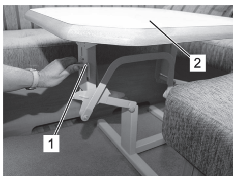
Afb. 153: tafel met heftafeldraagconstructie
